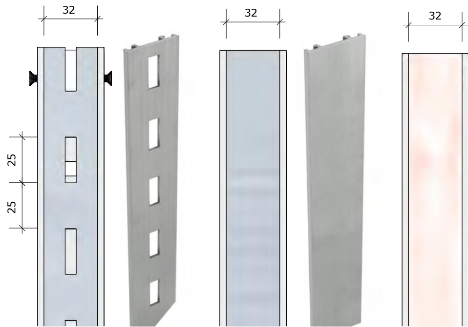
Fugenprofil, gelocht 3m 505.1.03
