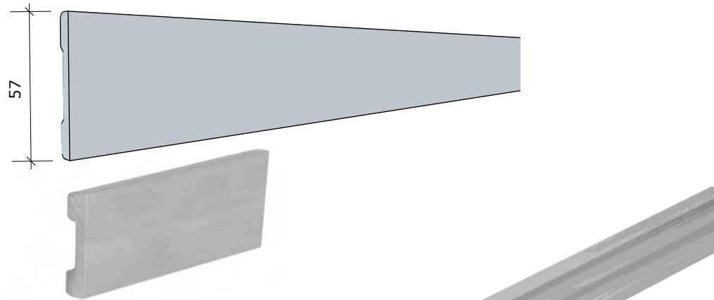
Fugenprofil, horizontal 3m 506.1.03
