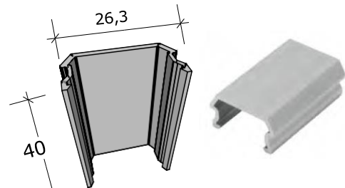
Fugenprofilsicherung 512.1.01
